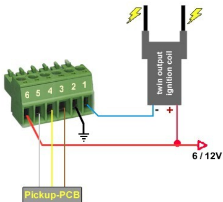
Anschlußdiagramm mit einer 6 V-Doppelzündspule.
