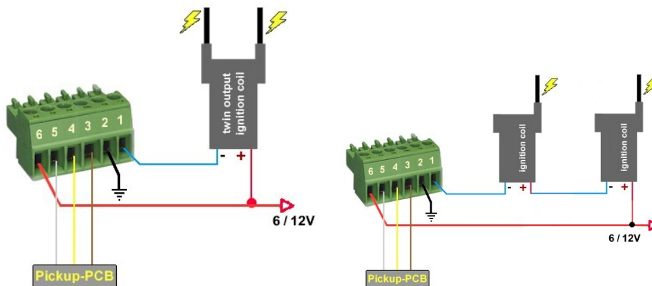
Anschlußdiagramm mit einer 12 V-Doppelzündspule.
