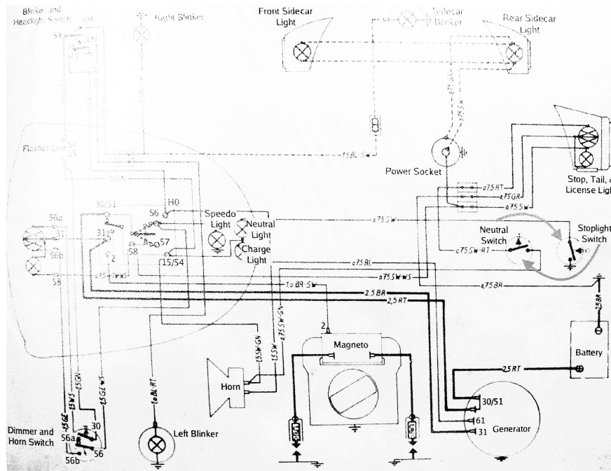
Abbildung 2 Originalschaltplan von der R69S.
