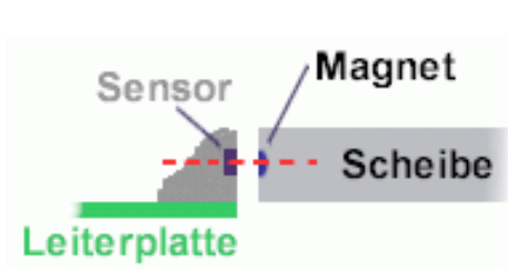
Abbildung 4 Korrekte Ausrichtung von Magnetring und Sensor.
