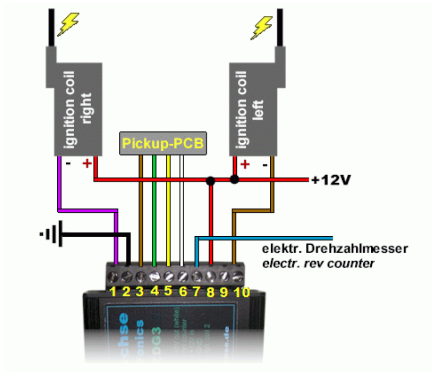
Anschlusschema der Zündung bei Motoplat-Ersatz
