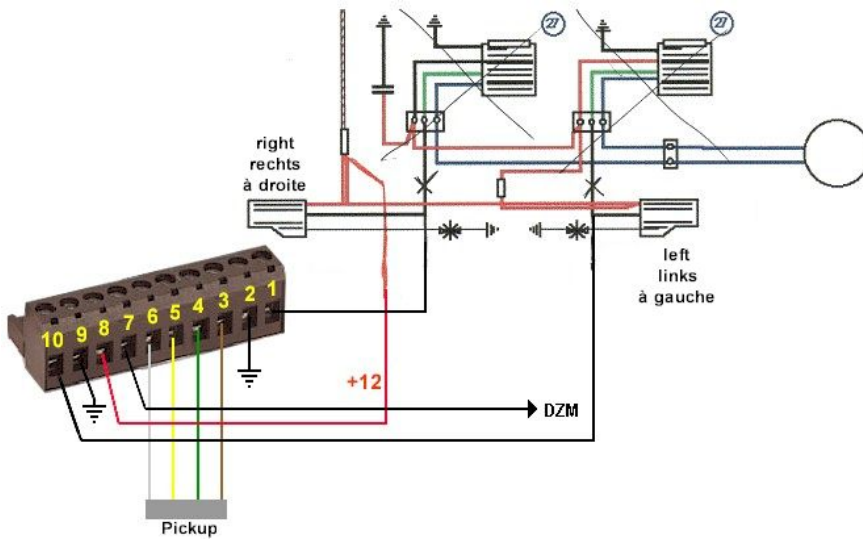
Anschlusschema der Zündung bei Kontakt-Ersatz
