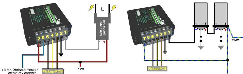
Anschlußdiagramm mit einer 12 V-Doppelzündspule.
