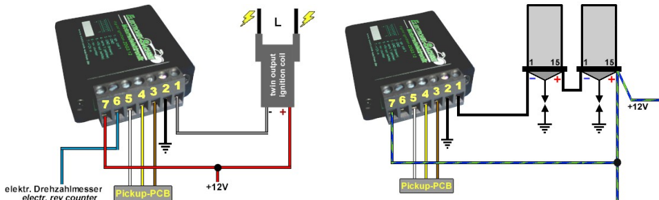
Anschlußdiagramm mit einer 12 V-Doppelzündspule.
