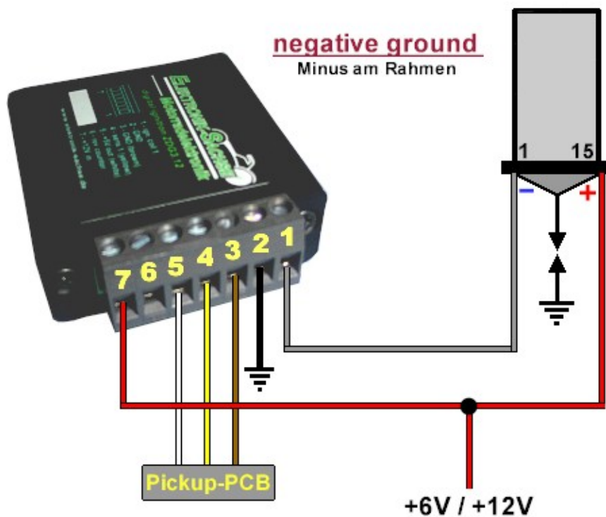
Generelles Anschlussschema
