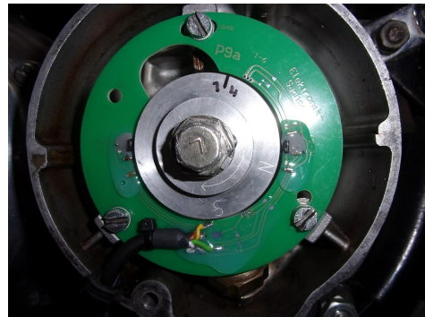
Abbildung 2 Montage des neuen Pickups, Mitnehmers und des Magnetringes. Die Madenschrauben im Magnetring noch nicht anziehen.
