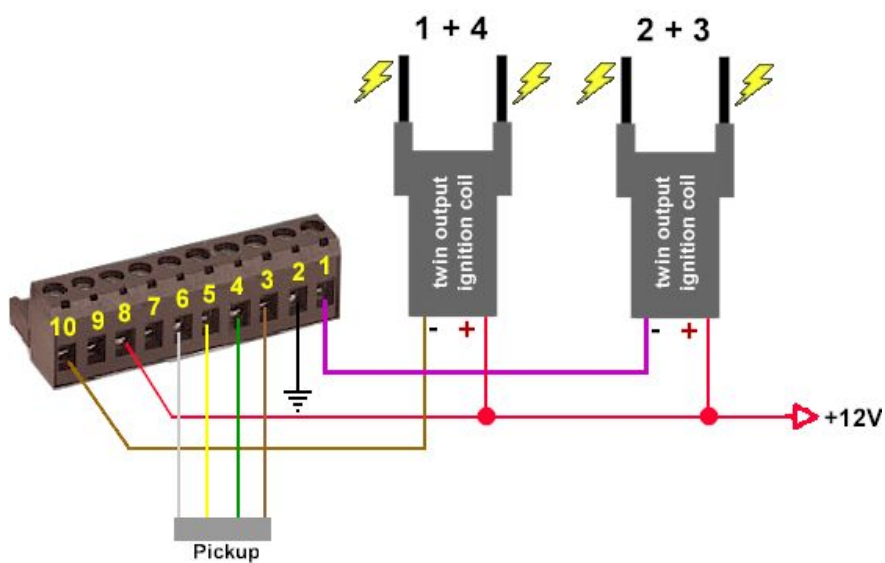
Abbildung 4 Anschlußschema
