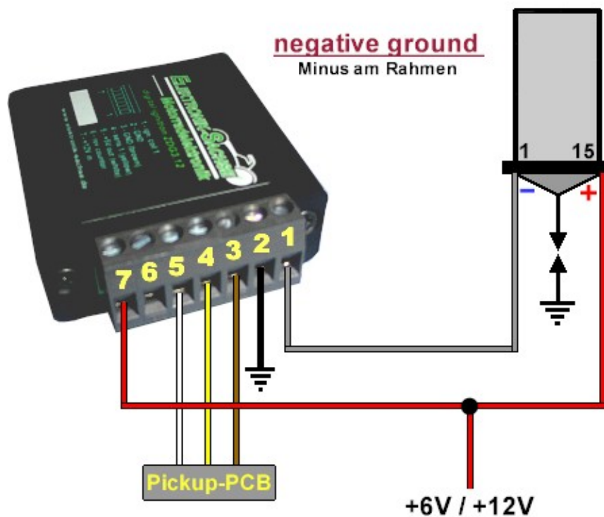
Generelles Anschlussschema
