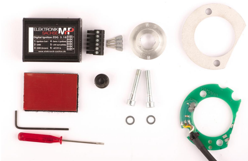
Abbildung 1 Lieferumfang
