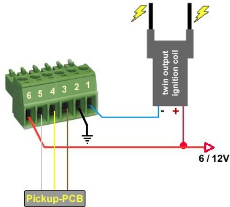
Abbildung 3 Anschlußschema
