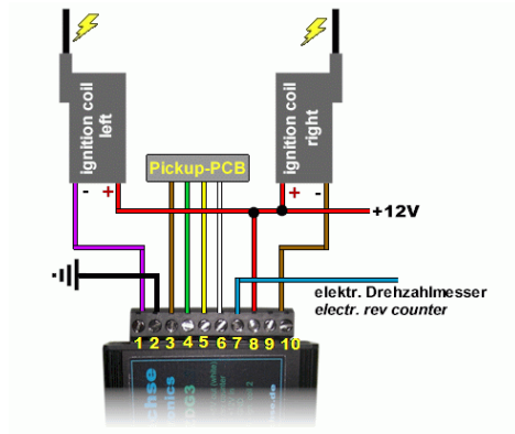
Elektrischer Anschluss der Zündung
