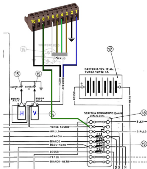
Abbildung 4 Anschluß im Stromlaufplan.
