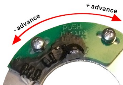
Abbildung 7 Feineinstellung des Versatzes der Frühzündung zwischen den beiden Zylindern.
