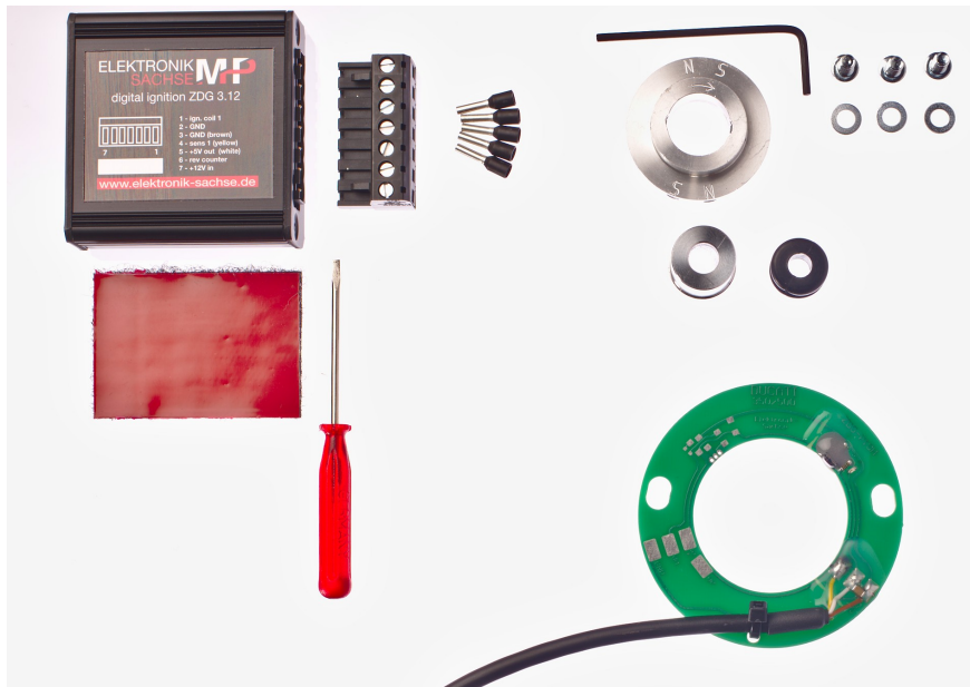
Abbildung 1 Lieferumfang
