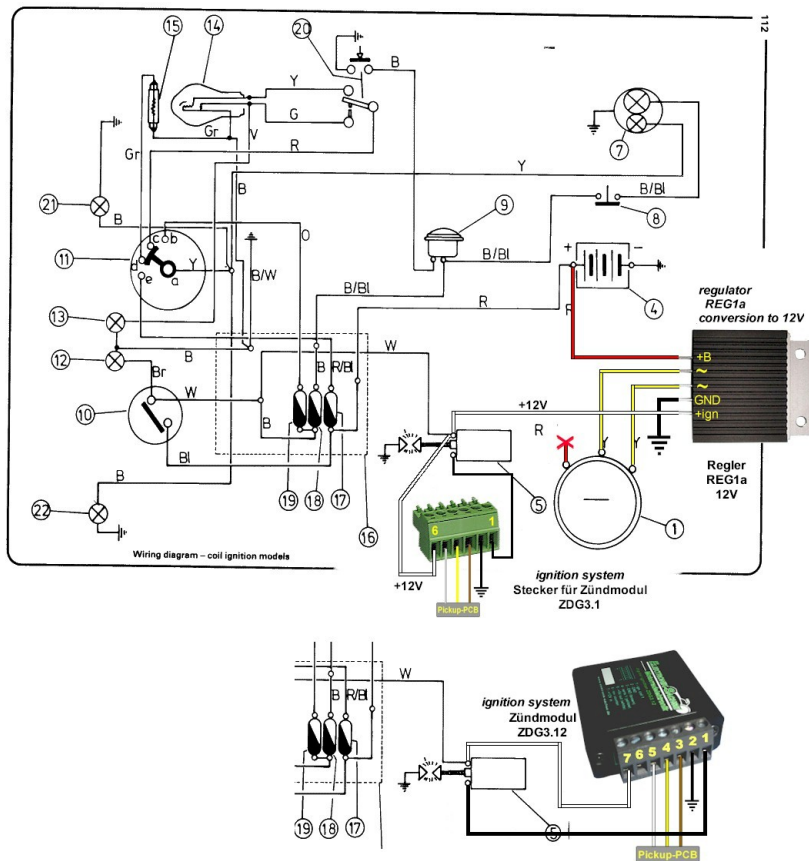
Elektrischer Anschluss der Zündung
