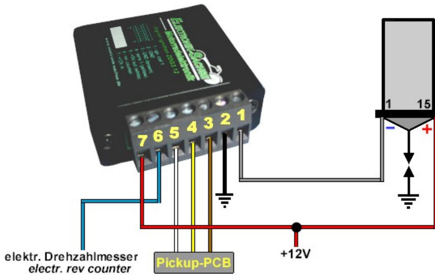
Abbildung 2 Anschlußschema
