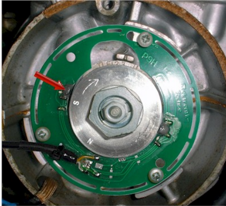
Abbildung 7 Auf diesem Sensor wird die Grundeinstellung gemacht.
