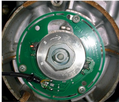
Abbildung 7 Die LED geht an, wenn der S-Magnet am Sensor vorbeiläuft.
