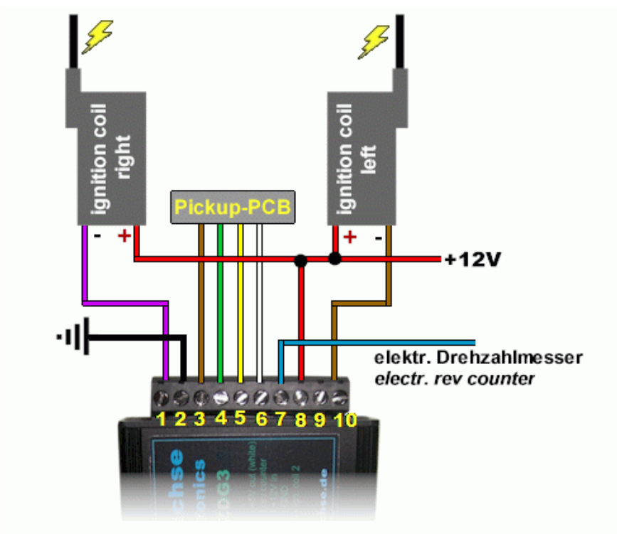
Abbildung 4 Anschluß mit zwei Einzelspulen (ZDG 3.23).
