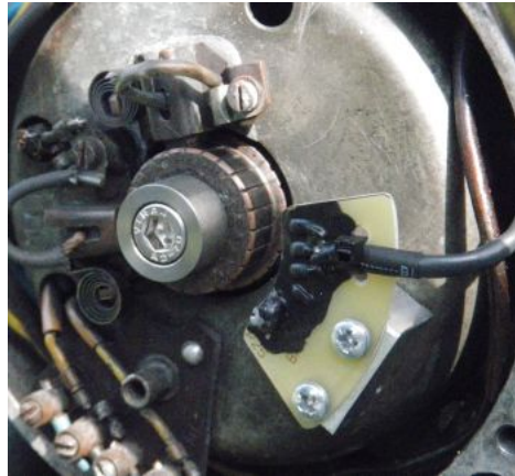
Die Rotormittelschraube entfernen und durch die mitgelieferte Inbusschraube und dem Mitnehmer ersetzen.
