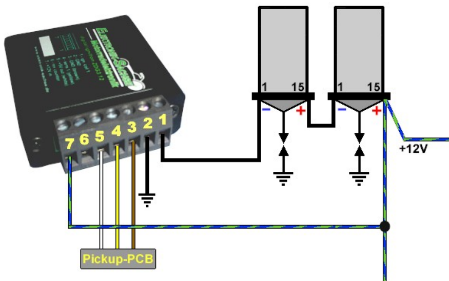
Elektrischer Anschluss der Zündung (originale Beschaltung mit zwei 6 V-Zündspulen in Reihe)
