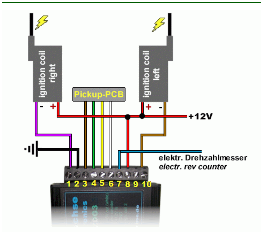
Elektrischer Anschluss der Zündung mit zwei 12V-Zündspulen.
